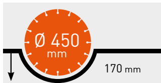
MAX. SCHNITTIEFE
